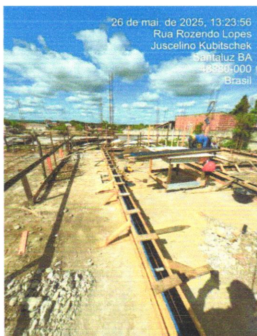
AMARRAÇÃO DE VIGAS E PILARES
